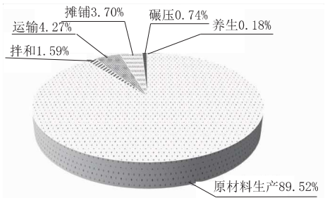
图 5 水稳基层 / 底基层施工各阶段碳排放量百分比
