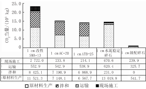
图 8 沥青路面各单位结构层碳排放量对比
