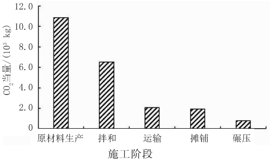
图 6 级配碎石垫层施工各阶段碳排放量
