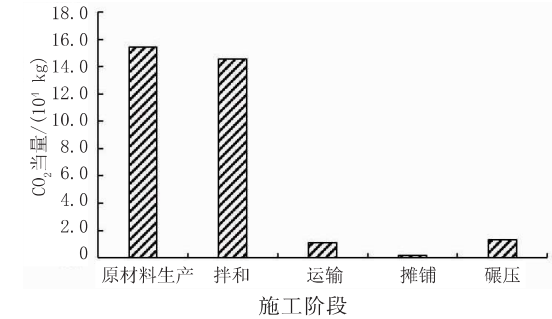
图 2 沥青面层施工各阶段碳排放量
