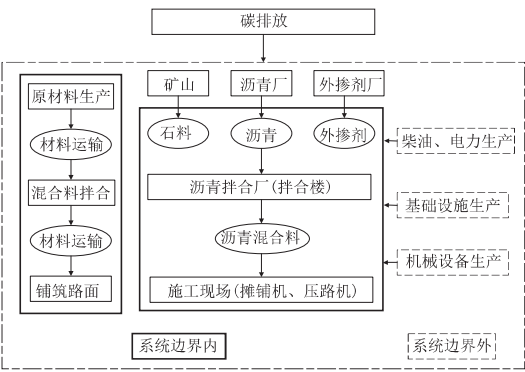
图 1 沥青路面施工期碳排放计量系统边界
