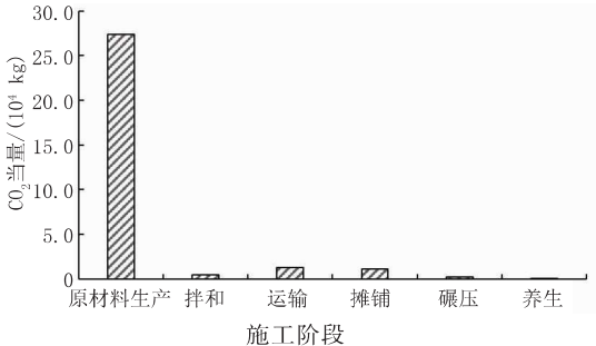
图 4 水稳基层 / 底基层施工各阶段碳排放量
