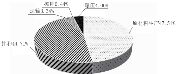
图 3 沥青面层施工各阶段碳排放量百分比
