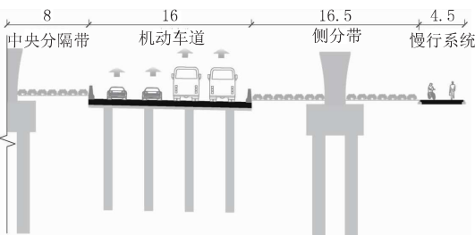
图2 右半幅标准横断面设计图(单位:m)
