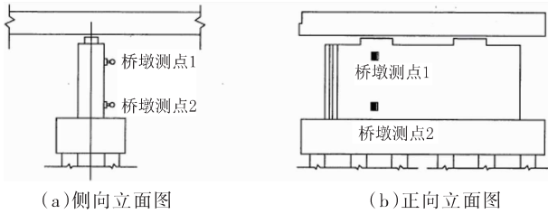
图 3 监测点布置示意图
