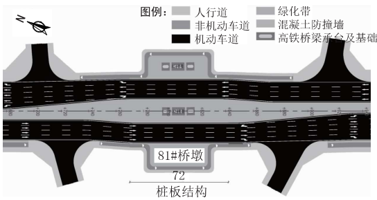
图1 整体设计方案图(单位:m)
